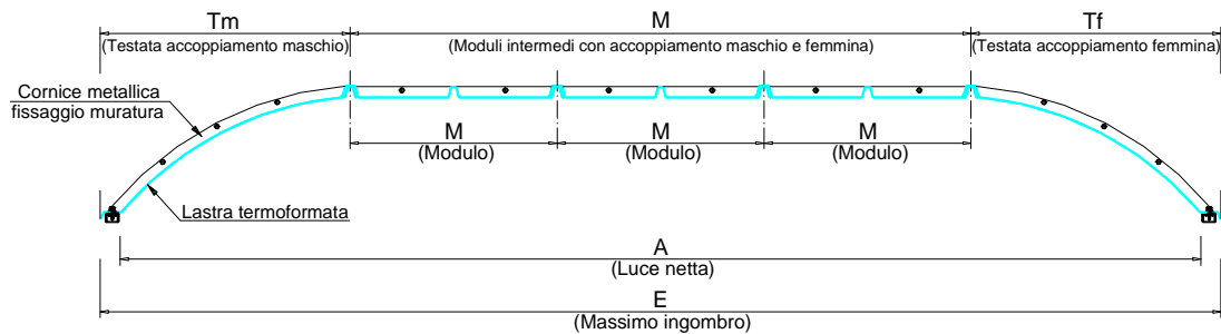
SEZIONE LONGITUDINALE
