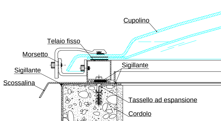
PARTICOLARE DI UN CUPOLINO COMPLETO DI TELAIO FISSO E SCOSSALINA (OPZIONALI)
