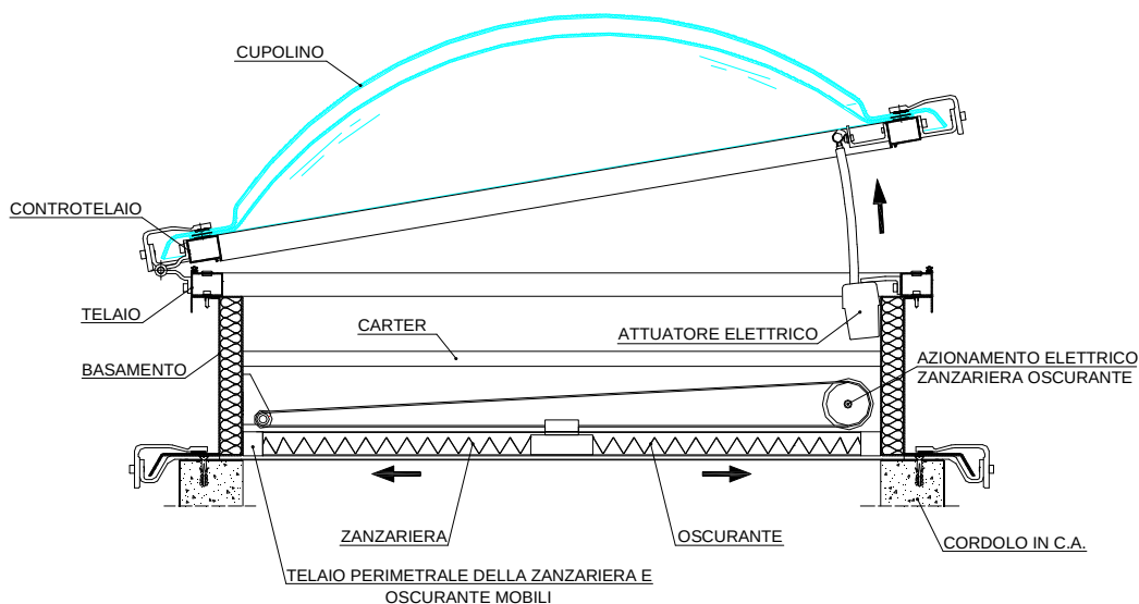
CUPOLINO A DOPPIA PARETE APRIBILE ELETTRICAMENTE CON BASAMENTO E OSCURANTE-ZANZARIERA AZIONATI ELETTRICAMENTE
